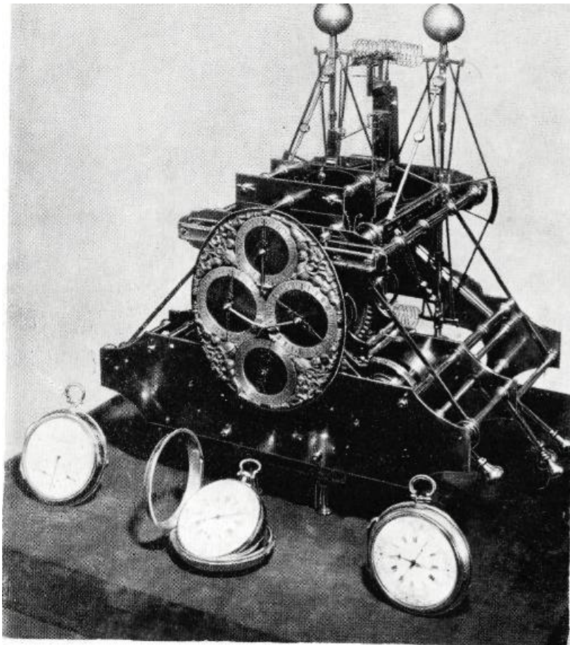
Морской хронометр. 1735 г.
